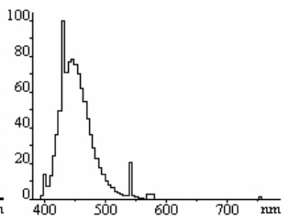
TLD 18 – światło niebieskie (blue light)
