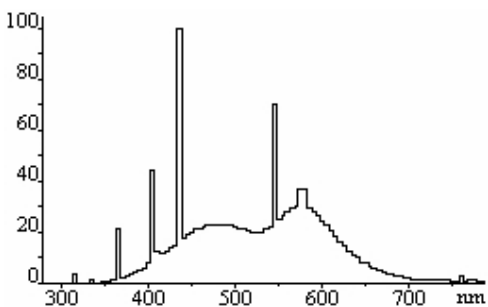
TLD 54 – światło dzienne (daylight)
