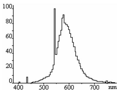
TLD 16 – światło żółte (yellow light)
