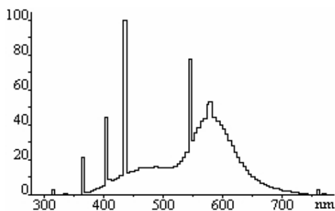
TLD 33 – światło białe (white light)
